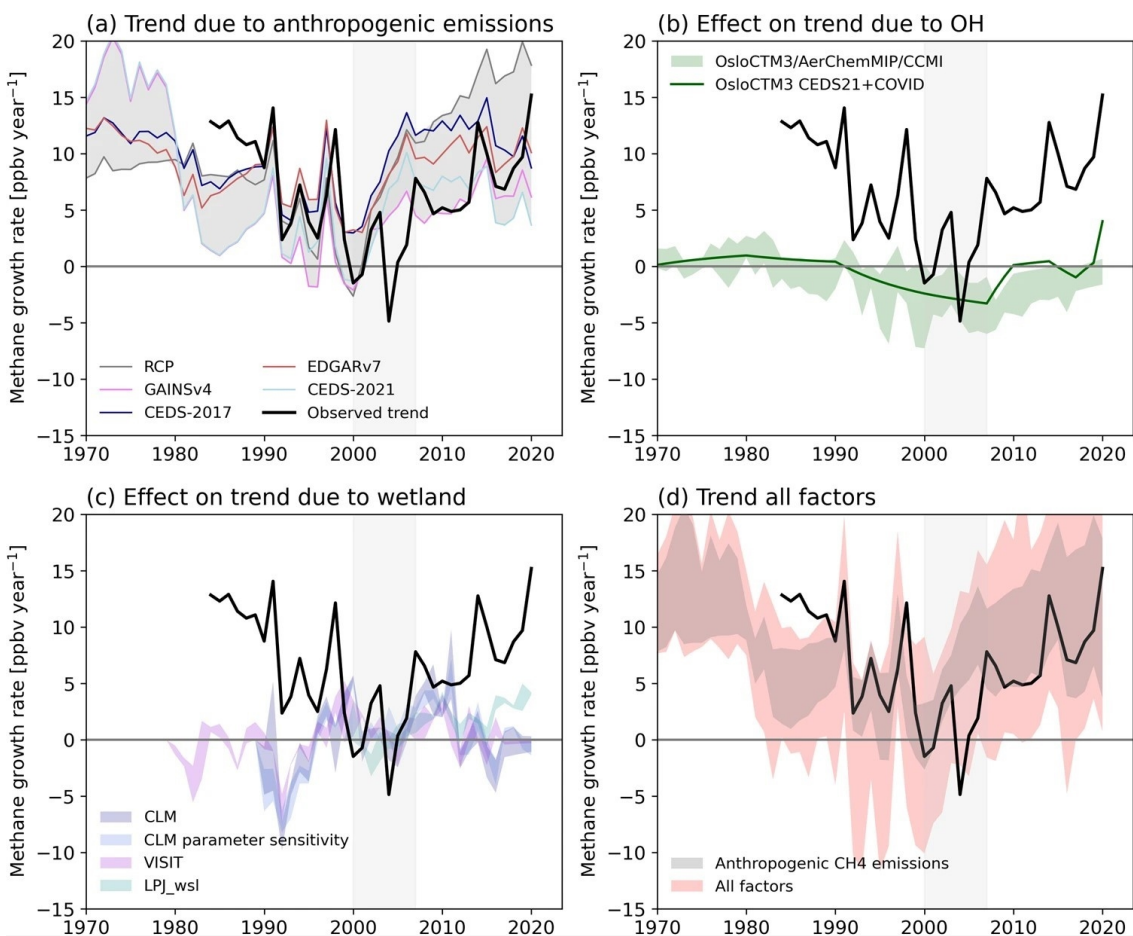
Tốc độ tăng methane khí quyển qua quan sát và tính toán [1]
